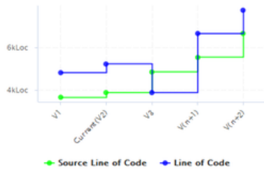
STEP
