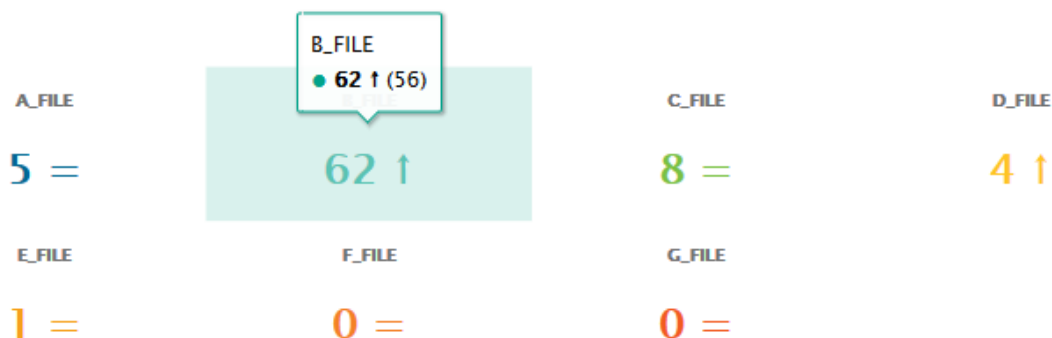
Text Values
