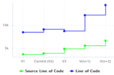
STACKED_STEP
