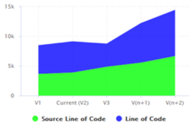
STACKED_AREA
