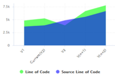
AREA
