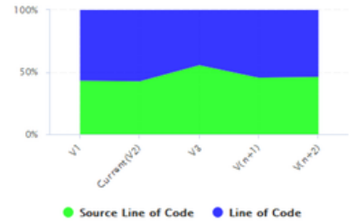
STACKED_AREA_100
