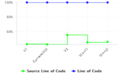
STACKED_STEP_100
